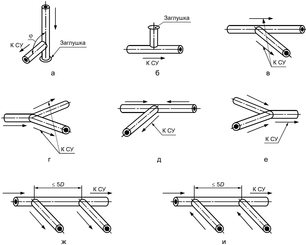
Рисунок А.2 — Тройники
